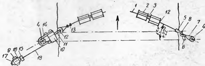
Рис. 3. Одногирляндная ГЭС (мощностью до 5 квт) на поперечных турбинах.
