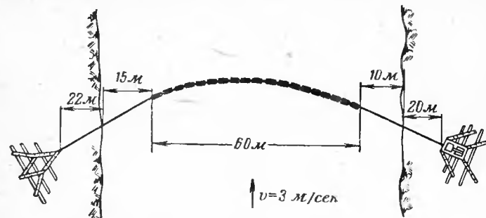
Рис. 20. Типовая схема установленной гирлянды с разметкой по створу ( D_{гирл} = 0,25 ; L_{гирл} = 60 \text{ м} ; N = 40 \text{ квт} ; береговые опоры подсыпаны камнем \sim 30 \text{ см} ).
