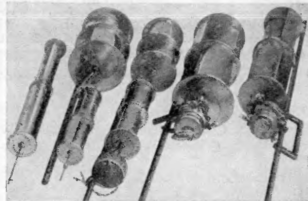
Рис. 26. Набор опытных образцов установок на поперечных турбинах, закрепленных на жестких осях.
