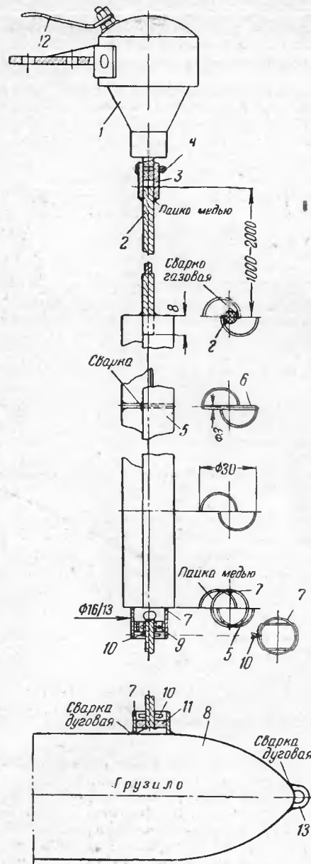
Рис. 31. Гидророторная переносная установка для освещения на ходу барж, катеров и рыболовецких баркасов.
