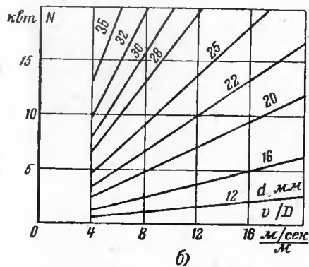
Рис. 19. Графики подбора тросовых трансмиссий (при \sigma_B = 3,5-7 \text{ кГ}/\text{мм}^2 ).
