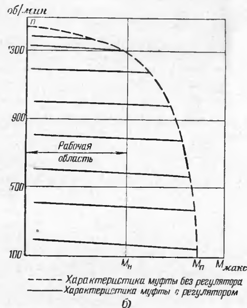
Рис. 24. Образцы характеристик муфт скольжения с регулятором скорости.
