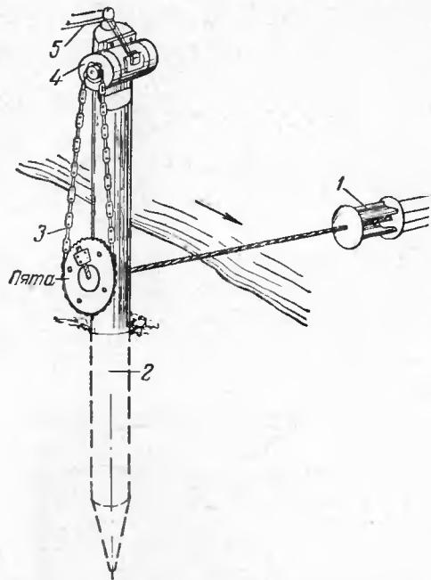
Рис. 15. Генераторная опора свайного типа. 1—гирлянда; 2—свая; 3—передача цепью Галля; 4—генератор; 5—проводка к потребителю.
