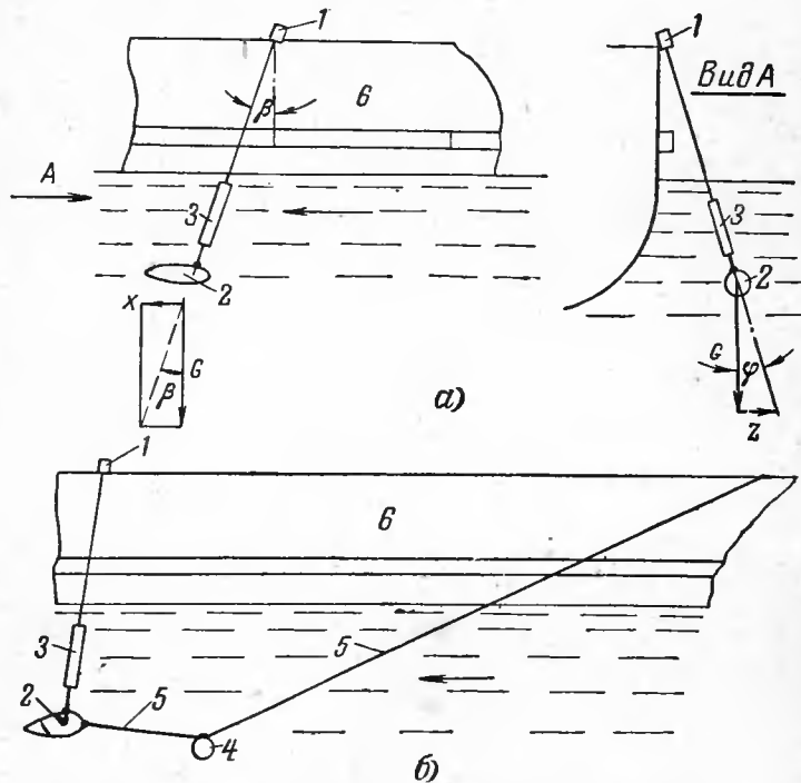
Рис. 32. Схема расположения забортных установок. 1 — генератор; 2 — грузило; 3 — турбина; 4 — оттягивающее грузило; 5 — натяжной шнур; 6 — корпус баржи или судна.
