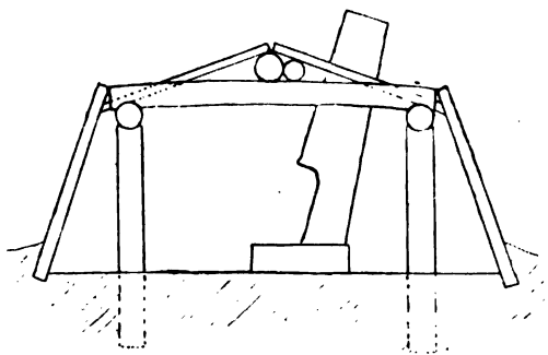
Рис. 66. Остовъ юрты.
